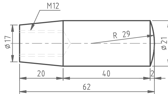
⑪ Handvat
